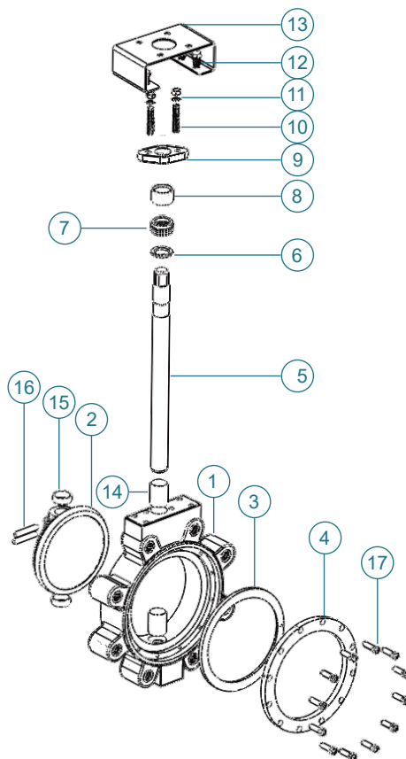
Lug type
